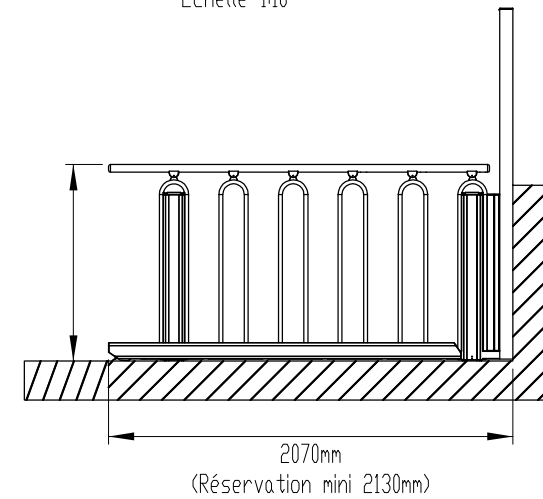
Détail A Echelle 1:10
